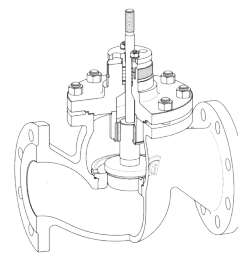
Reglerventil med övre kägelstyrning
