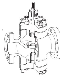
Reglerventil med övre kägelstyrning
